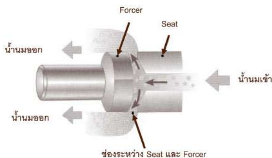
ภาพที่ 78 : การทำงานของเครื่องโฮโมจิไนส์ขณะใช้ความดันสูงอัดน้ำมันผ่านช่องว่าง
